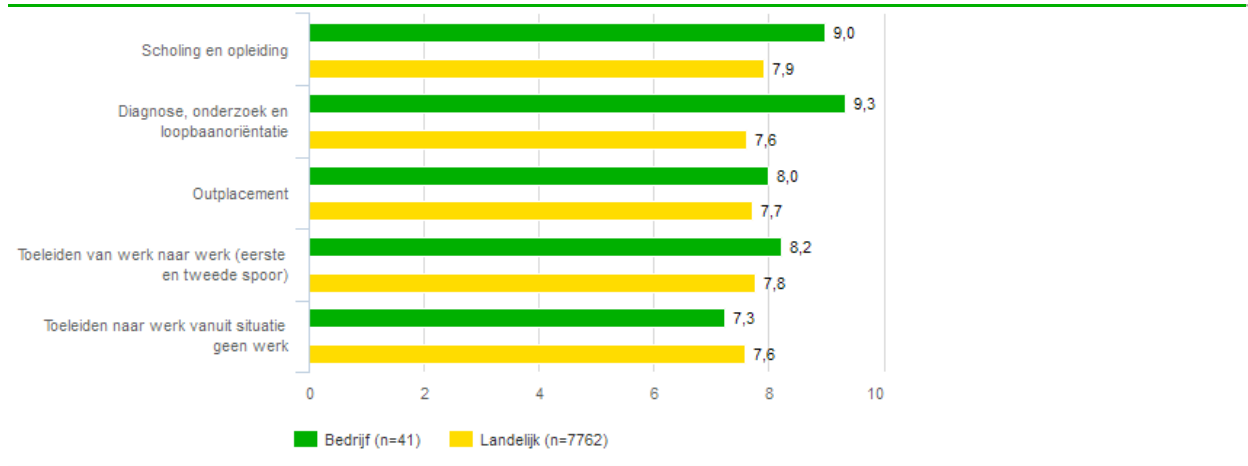
fig. 3.1 Gemiddeld rapportcijfer
