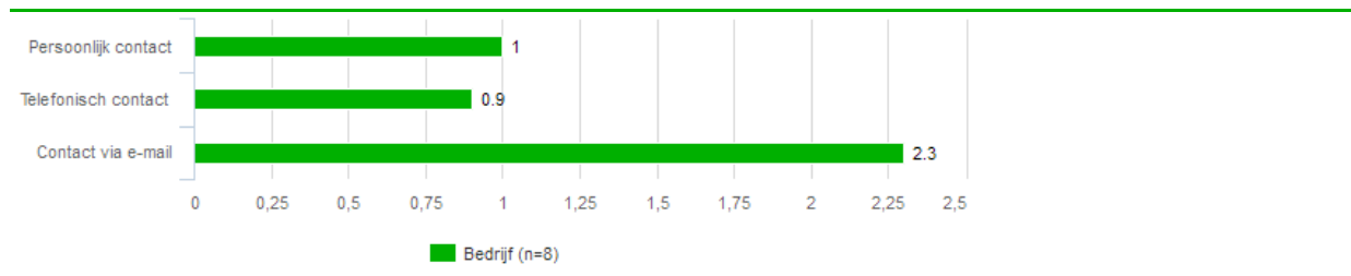
fig. 3.9 Hoe vaak heeft u contact gehad met Intraverte Reset BV? Geef hier een inschatting van hoe vaak u gemiddeld per maand contact had met medewerkers van Intraverte Reset BV
