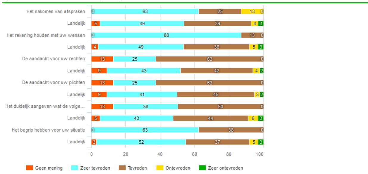
fig. 3.14 Hoe tevreden bent u over de begeleiding door Intraverte Reset BV?
