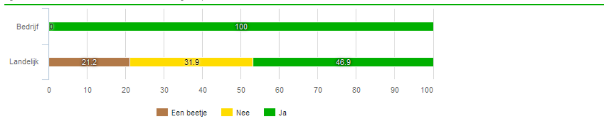
fig. 3.18 Heeft Intraverte Reset BV hier mee geholpen?
