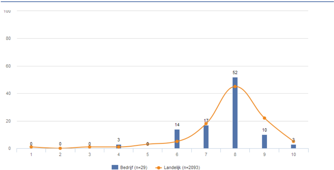
fig. 4.2 Spreiding rapportcijfers
